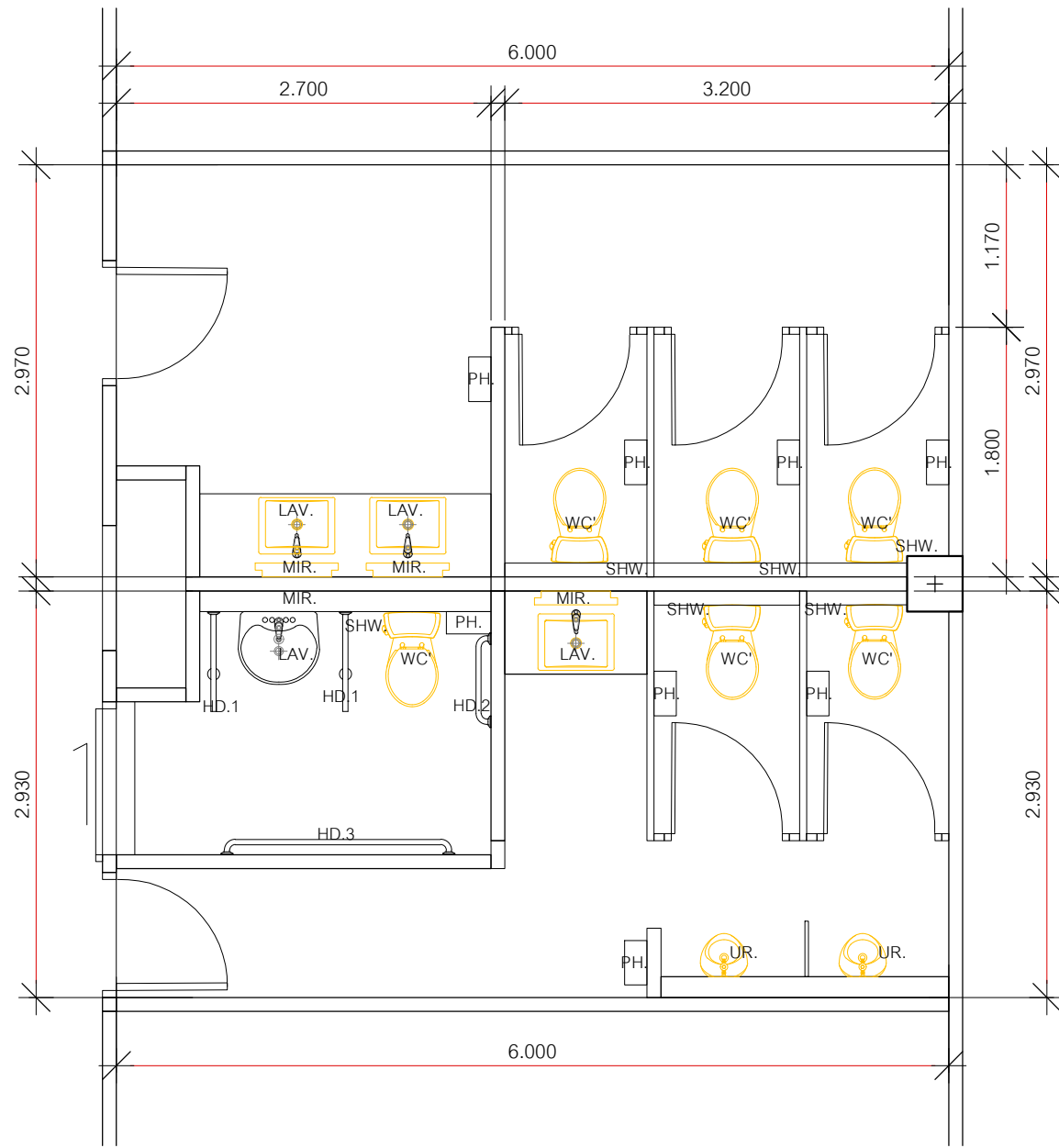
แบบแปลน สุขภัณฑ์และอุปกรณ์ SCALE A3 //1: 50
