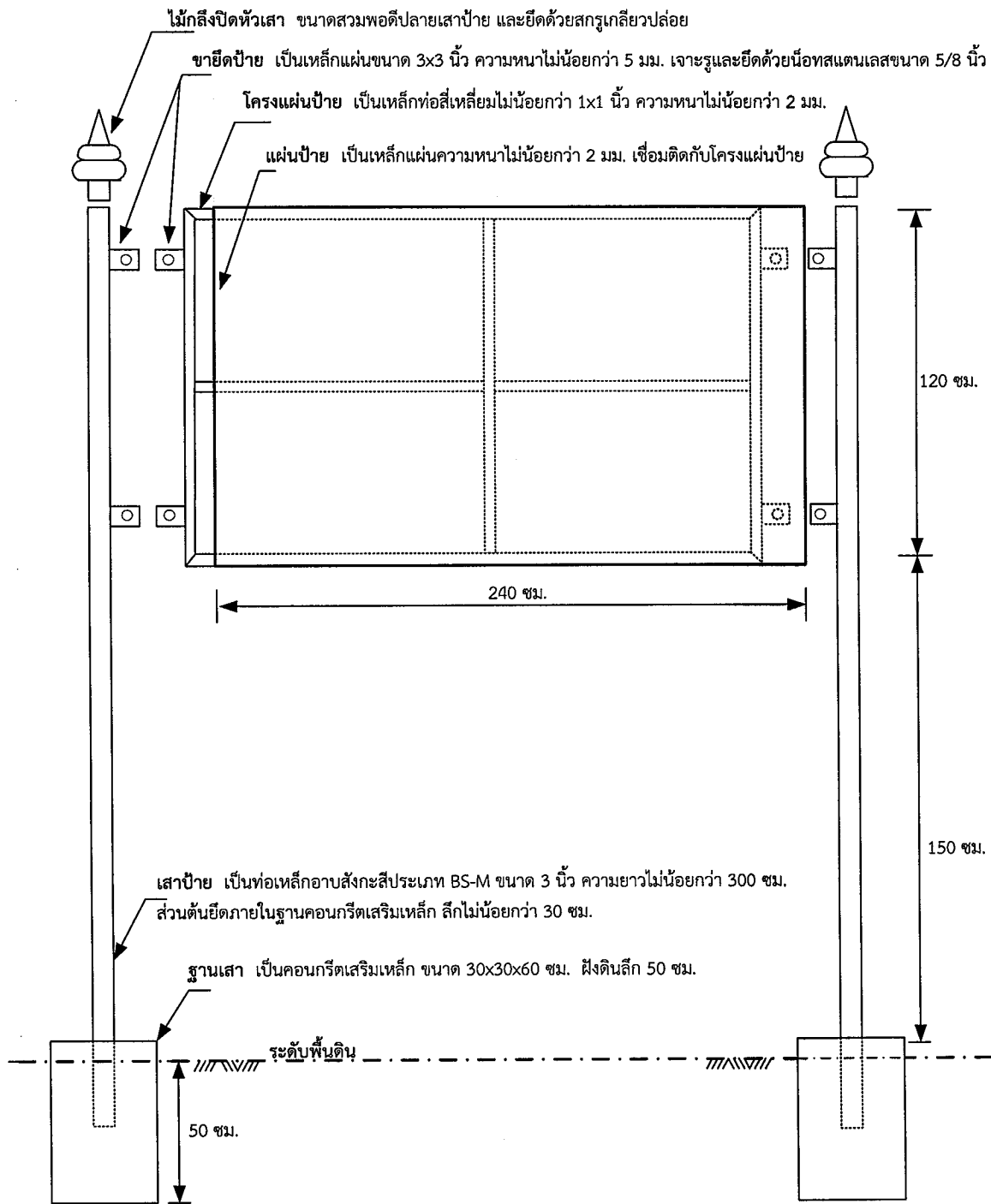
รูปที่ ๒ ลักษณะรูปแบบโครงสร้างป้ายชื่อโครงการ (หมายเหตุ รูปนี้ไม่ได้แสดงอัตราส่วน)
