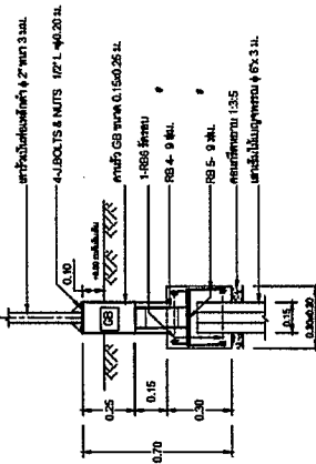
แบบขยายฐานราก F (แบบมีเสาเข็ม) มาตราส่วน 1:25
