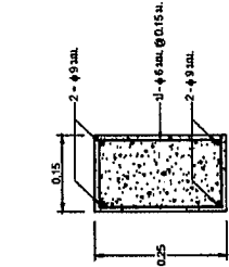
แบบขยายฐาน GB มาตราส่วน 1:10
