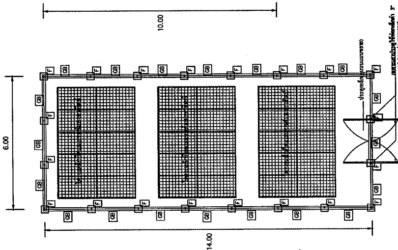
แปลนห้องเครื่องต้มน้ำ 7.5 kW มาตราส่วน 1:100
